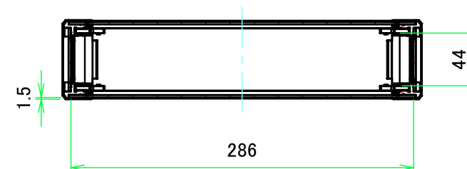
A-A ( 1:4.5 )
