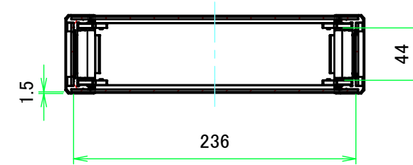
A-A ( 1:4.5 )
