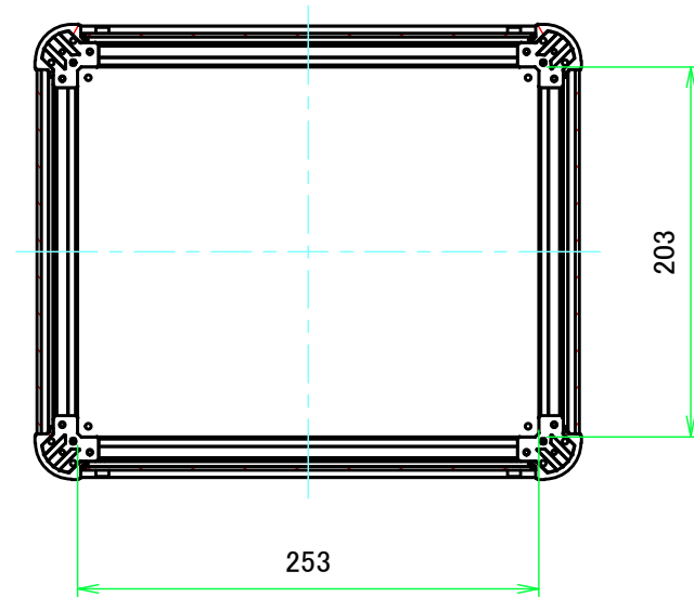
B-B ( 1:4.5 )
