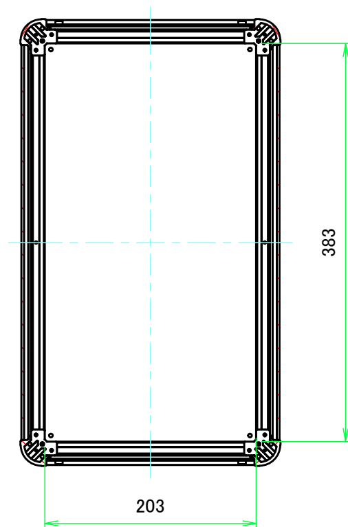
B-B ( 1:5 )
