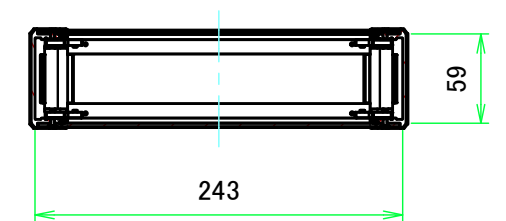
C-C ( 1:5 )
