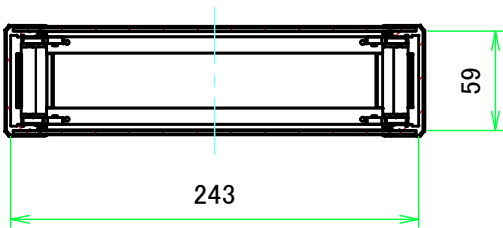
C-C ( 1:4.5 )
