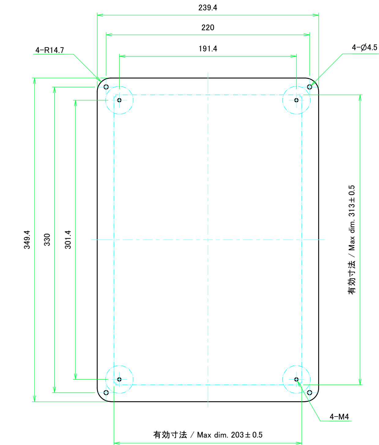
保護シート側 Surface protective film side
