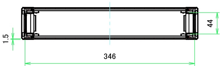
A-A ( 1:4.5 )
