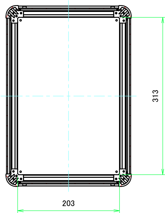
B-B ( 1:4.5 )
