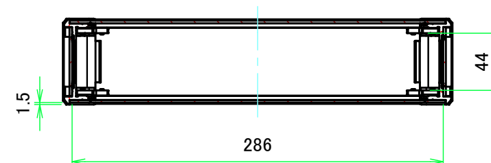
A-A ( 1:4 )
