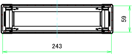
C-C ( 1:4 )
