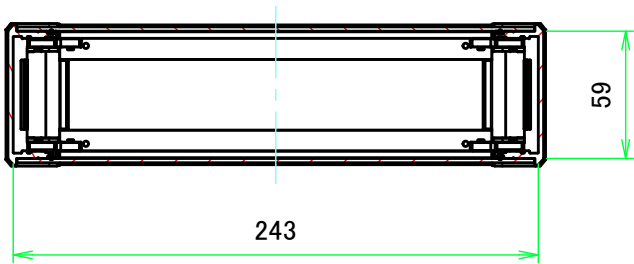
C-C ( 1:3.5 )
