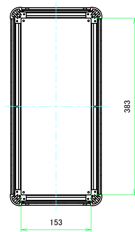
B-B ( 1:5 )
