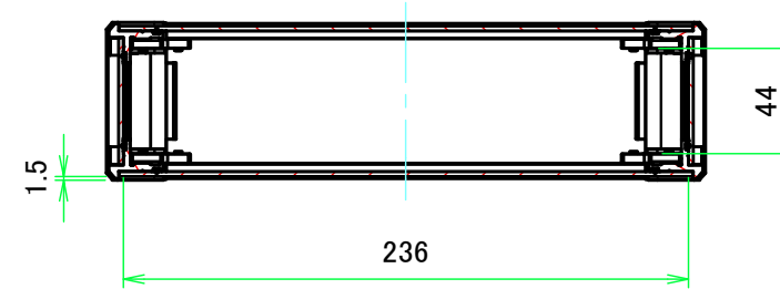
A-A ( 1:3.5 )
