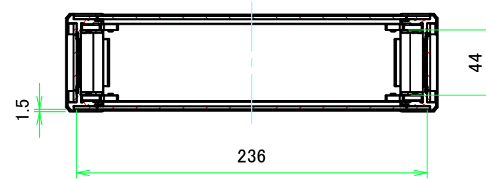
A-A ( 1:3.5 )
