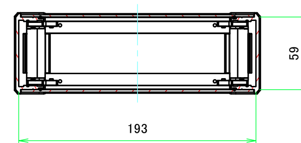
C-C ( 1:3 )
