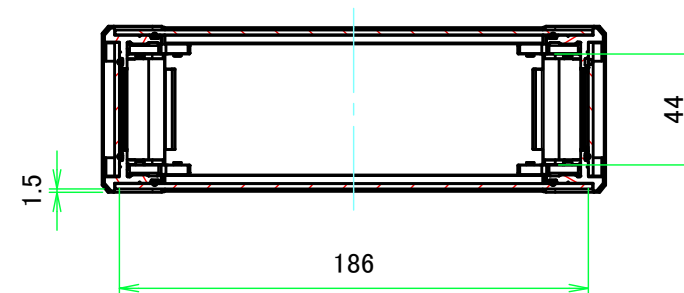
A-A ( 1:3 )
