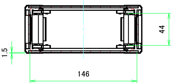
A-A ( 1:3 )
