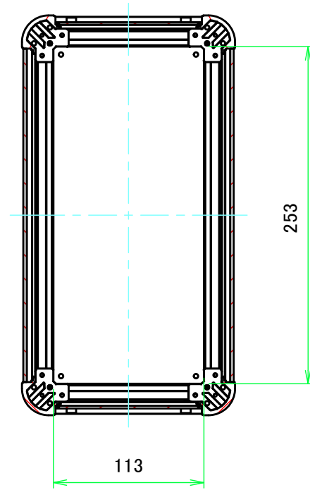
B-B ( 1:4 )
