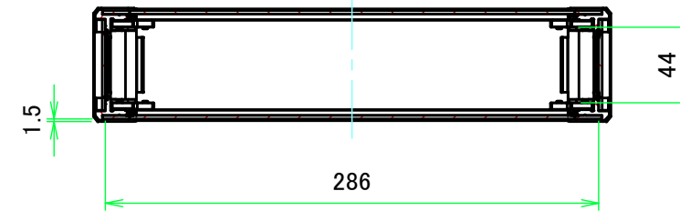
A-A ( 1:4 )
