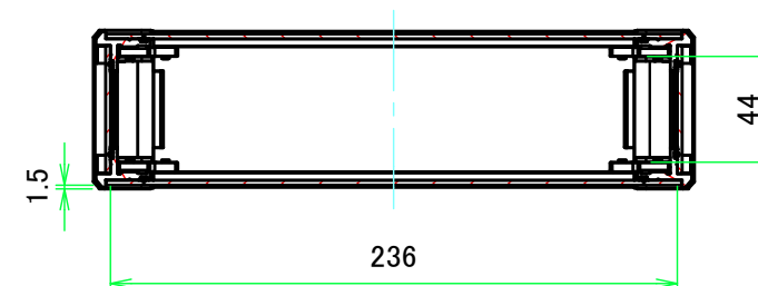
A-A ( 1:3.5 )
