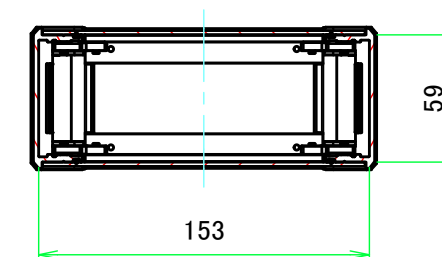
C-C ( 1:3.5 )
