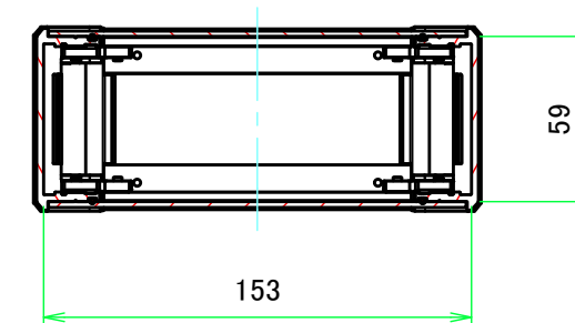
C-C ( 1:3 )
