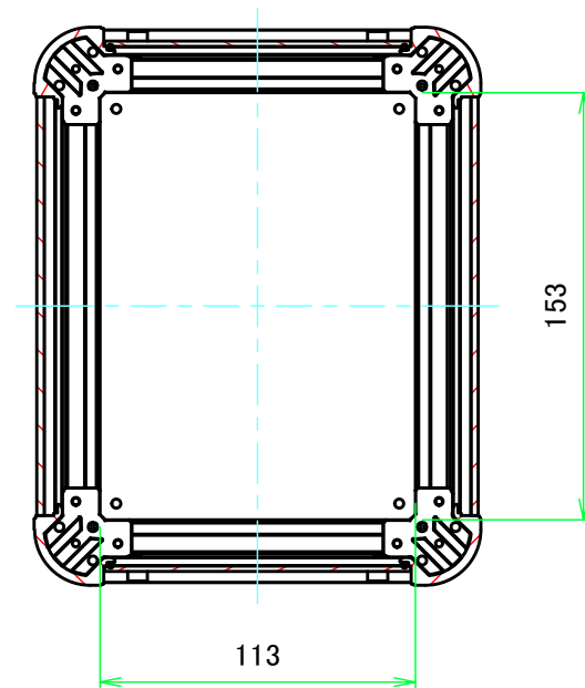
B-B ( 1:3 )
