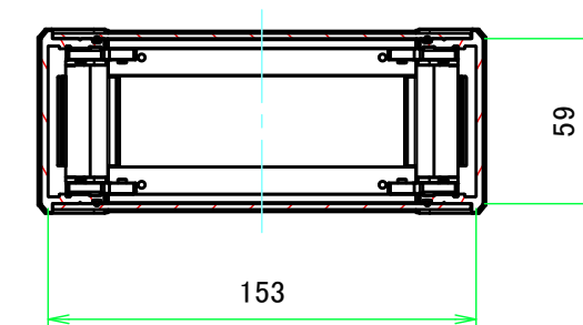
C-C ( 1:3 )
