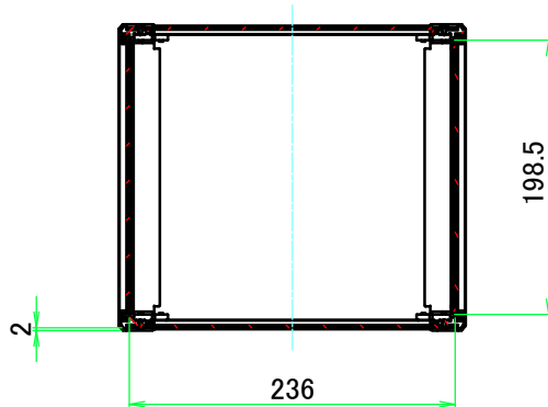
A-A ( 1 : 6 )
