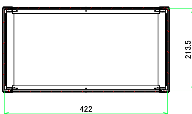
C-C ( 1 : 6 )
