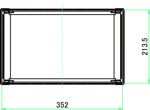
C-C ( 1 : 6.5 )
