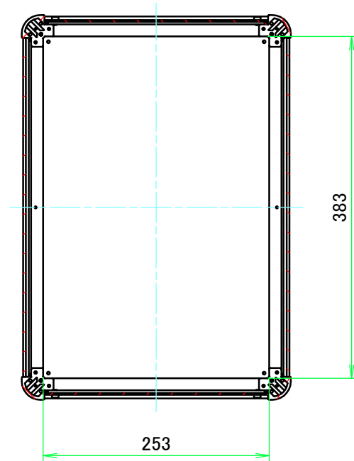
B-B ( 1 : 6 )
