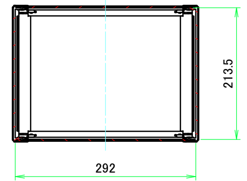
C-C ( 1 : 6 )
