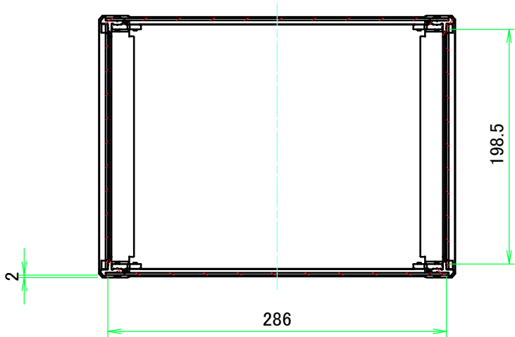
A-A ( 1 : 4.5 )
