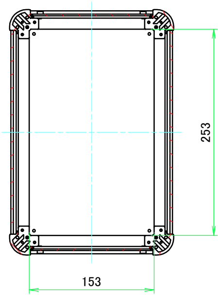
B-B ( 1 : 4.5 )
