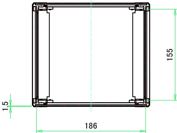
A-A ( 1 : 4 )
