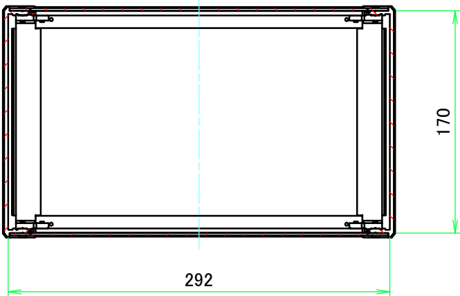
C-C ( 1 : 4 )
