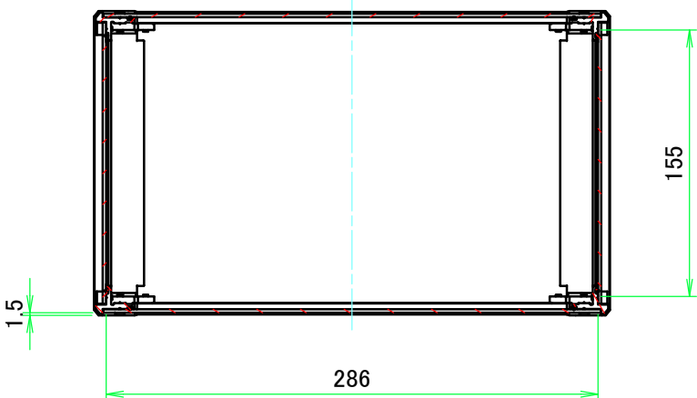
A-A ( 1 : 4 )
