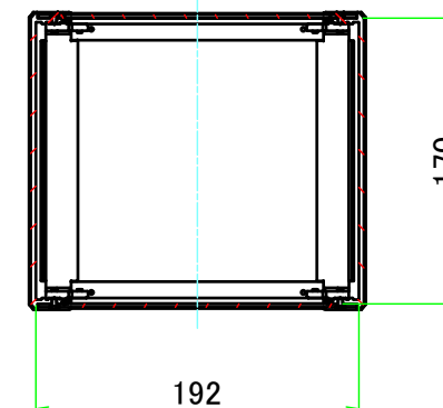
C-C ( 1 : 5 )
