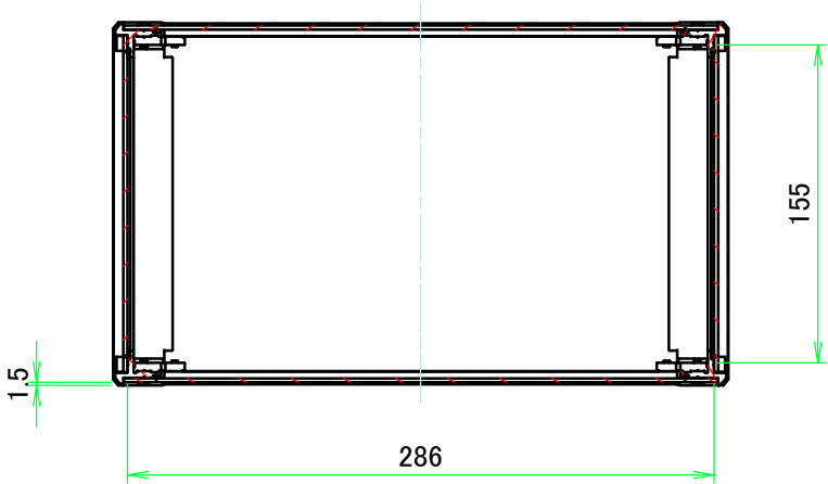
A-A ( 1 : 4 )
