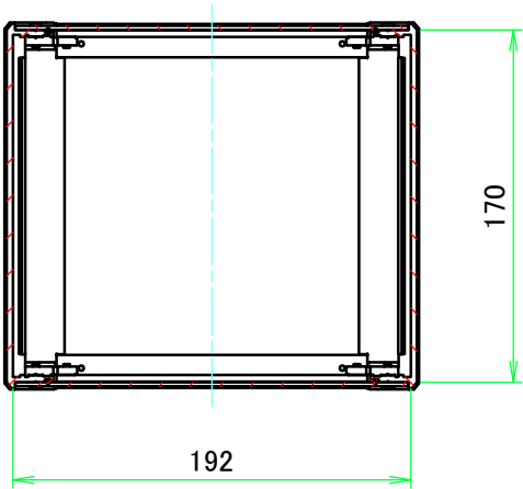
C-C ( 1 : 4 )
