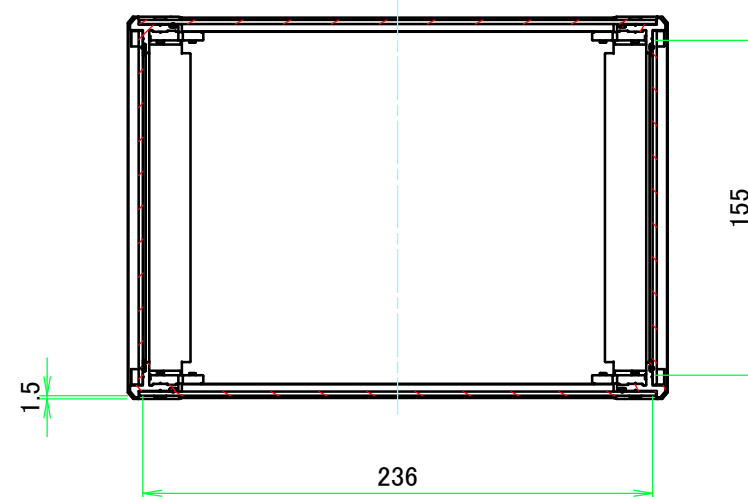
A-A ( 1 :3.5 )
