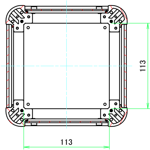
B-B ( 1 : 3 )
