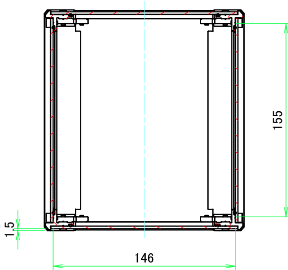
A-A ( 1 : 3 )
