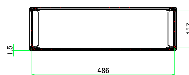
A-A ( 1 : 7.5 )
