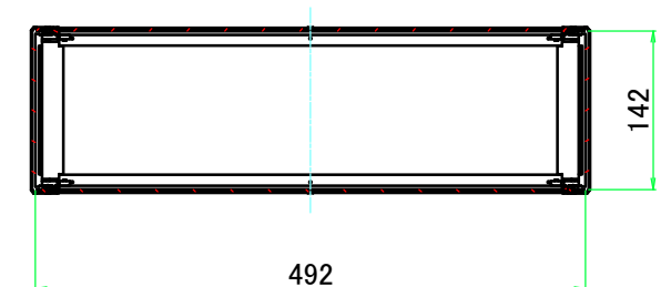
C-C ( 1 : 7.5 )
