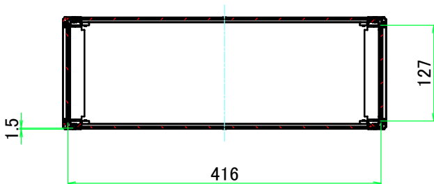
A-A ( 1 : 7 )
