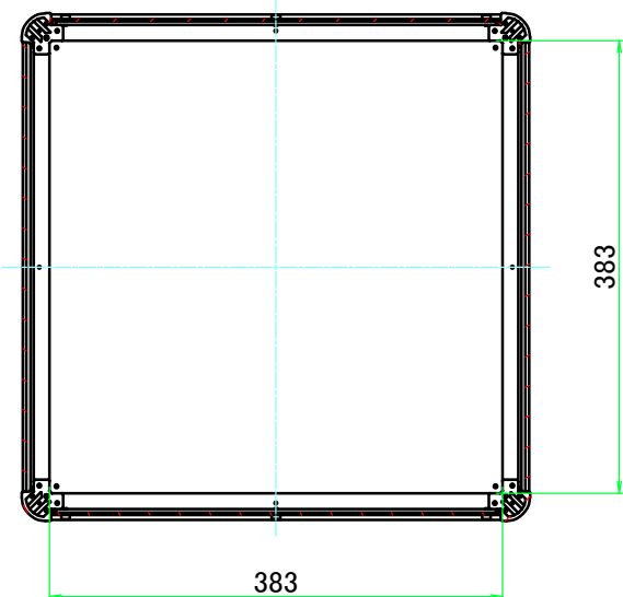
B-B ( 1 : 7 )
