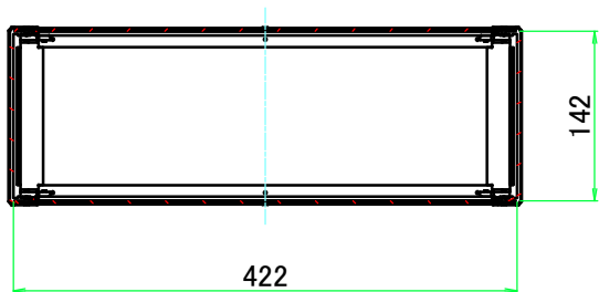
C-C ( 1 : 7 )
