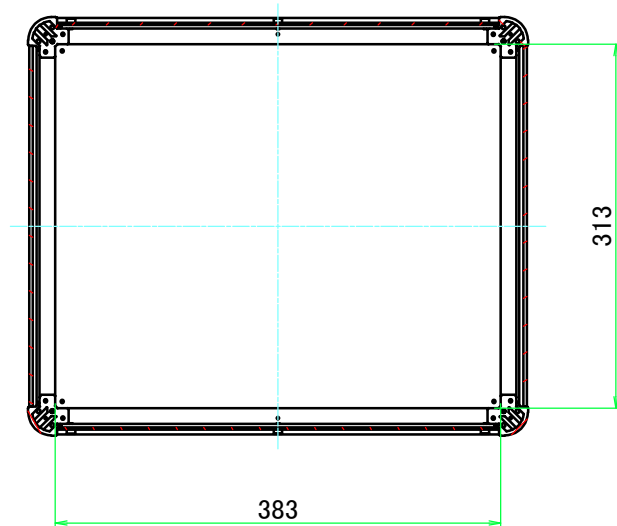
B-B ( 1 : 6.5 )
