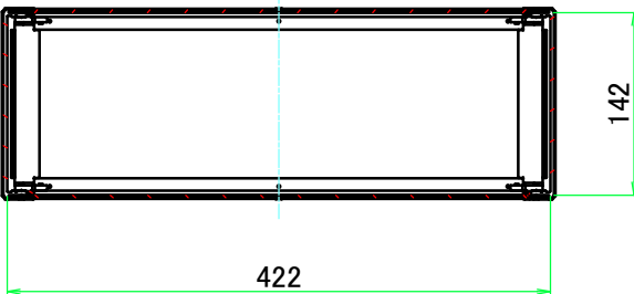
C-C ( 1 : 6.5 )
