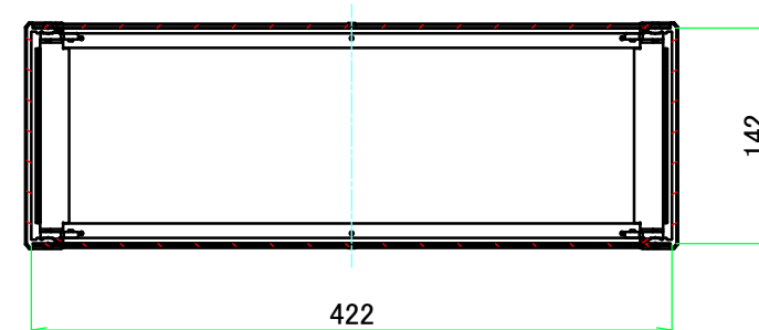
C-C ( 1 : 5.5 )
