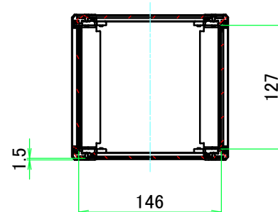
A-A ( 1 : 5.5 )
