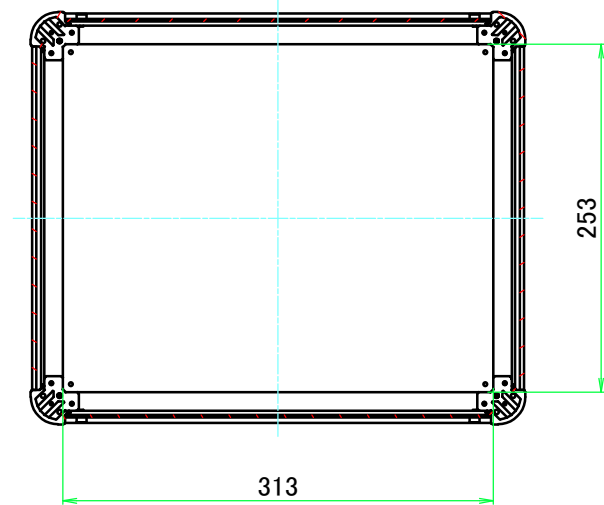
B-B ( 1 : 5.5 )
