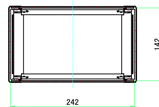
C-C ( 1 : 4.5 )
