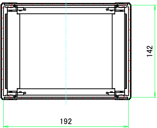
C-C ( 1 : 3.5 )
