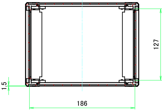
A-A ( 1 : 3.5 )
