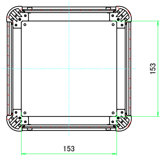
B-B ( 1 : 3.5 )
