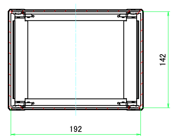
C-C ( 1 : 3.5 )
