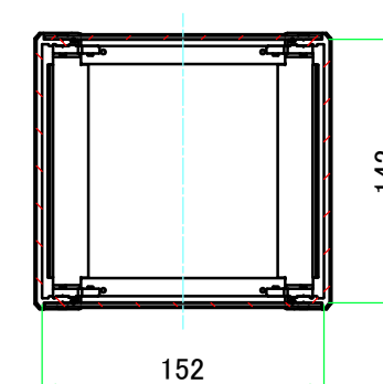
C-C ( 1 : 4.5 )
