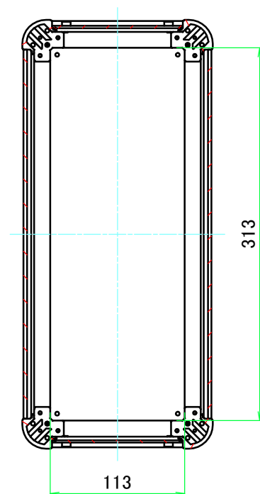
B-B ( 1 : 4.5 )
