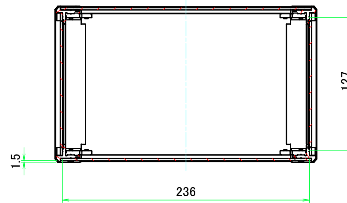
A-A ( 1 : 3.5 )
