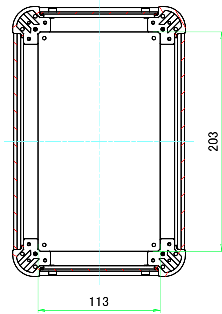
B-B ( 1 : 3.5 )
