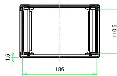
A-A (1:4)
