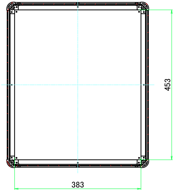
B-B ( 1 : 7 )
