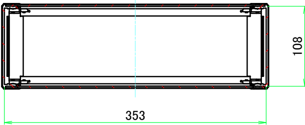
C-C ( 1 : 5 )
