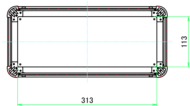
B-B ( 1 : 5 )
