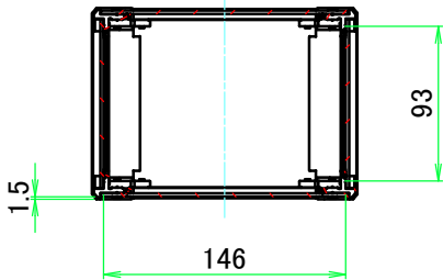
A-A ( 1 : 5 )
