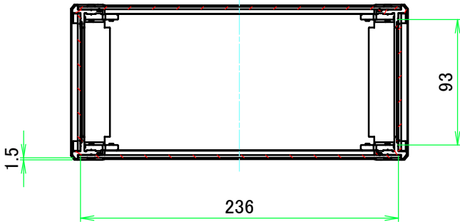
A-A ( 1 : 4 )
