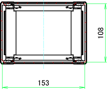
C-C ( 1 : 4 )
