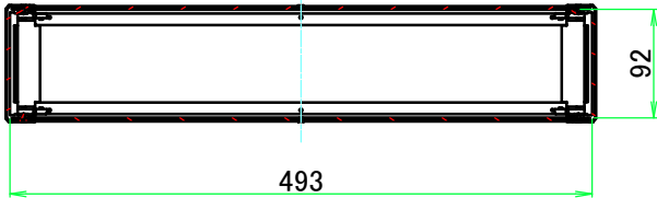
C-C ( 1 : 7 )
