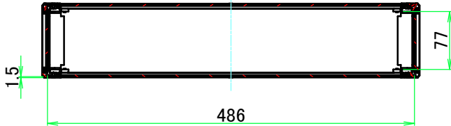
A-A ( 1 : 7 )
