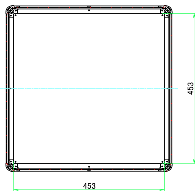
B-B ( 1 : 7 )
