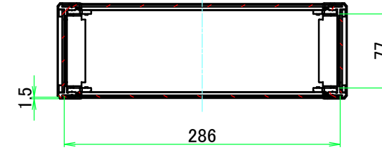
A-A ( 1 : 5.5 )
