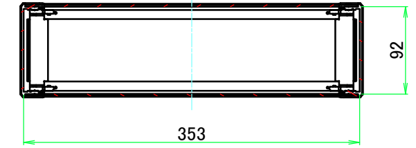
C-C ( 1 : 5.5 )
