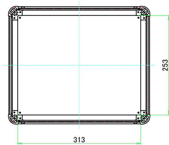
B-B ( 1 : 5.5 )
