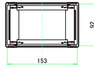
C-C ( 1 : 4 )
