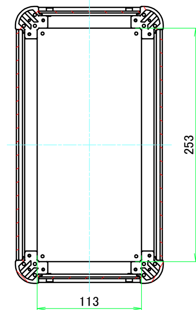
B-B ( 1 : 4 )
