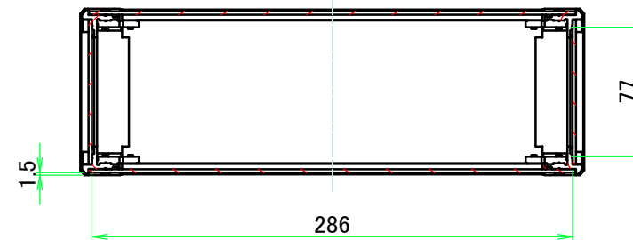
A-A ( 1 : 4 )
