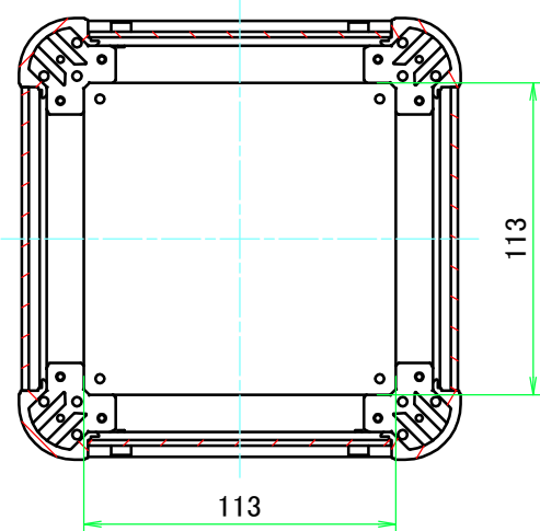
B-B ( 1 : 3 )
