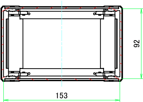
C-C ( 1 : 3 )
