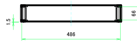
A-A (1:7.5)
