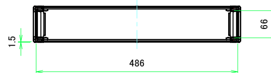
A-A (1:6.5)
