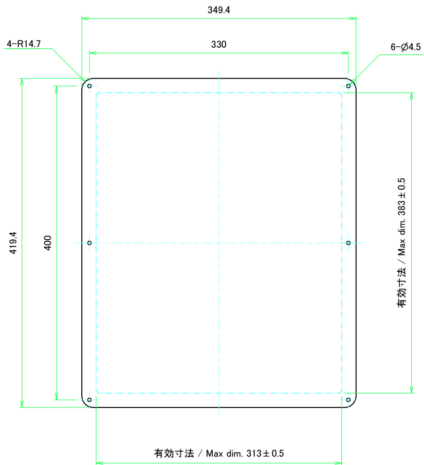
保護シート側 Surface protective film side
