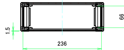
A-A (1:5)
