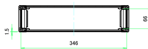
A-A (1:5)
