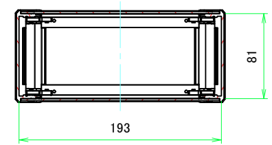
C-C (1:3.5)
